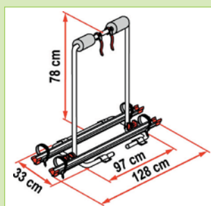
6503 Porte-vélos sur flèche s'adapte à toutes les remorques flèche en V. La partie supérieure pivote pour laisser l'accès à la porte avant ou pour placer plus facilement les vélos. Pour 2 vélos.
